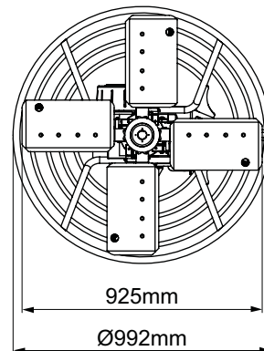
DIAMÈTRE DE LA TALOCHUEUSE & DIAMÈTRE DE L'ANNEAU
