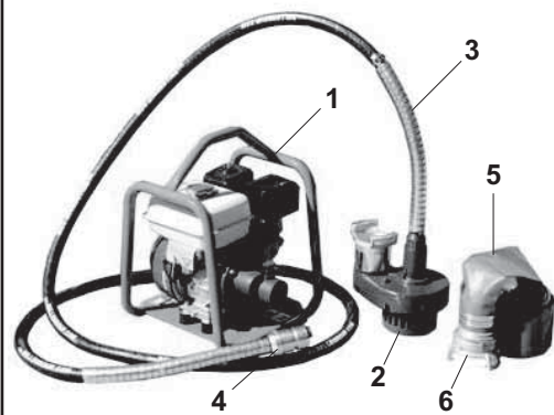
Bomba de Agua Sumergible (5M)
