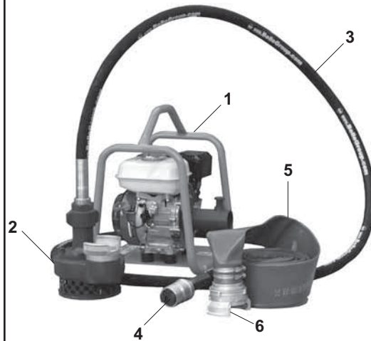
Versenkbare Pumpe (7M)
