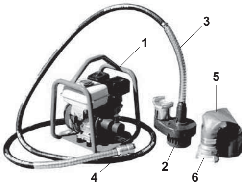
Versenkbare Pumpe (5M)
