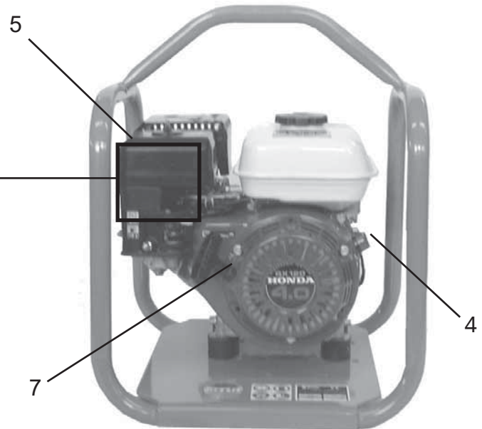
Brandstoftoevoerhendel
