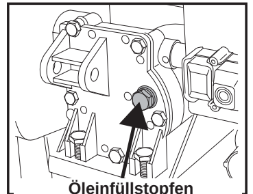
Getriebeöl-Einfüllposition
