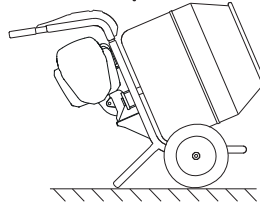
Getriebeöl-Einfüllposition
