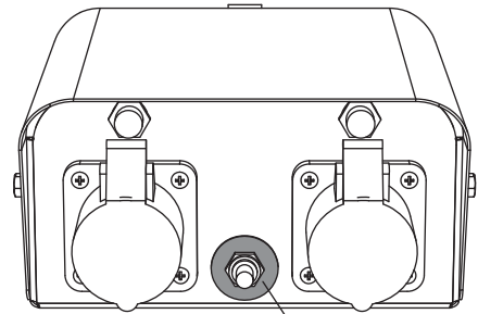
Vista delantera de la caja de conexiones
